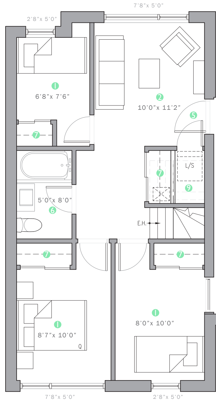
NIVEAU 3 (OPTION 2) - 642 PI.CA
