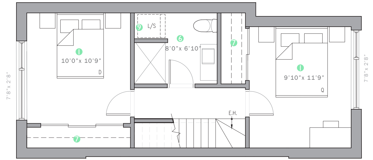
NIVEAU 0 - 540 PI.CA
